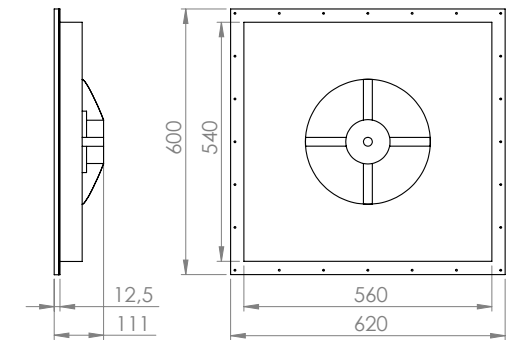
cerasonar 6062 sub
